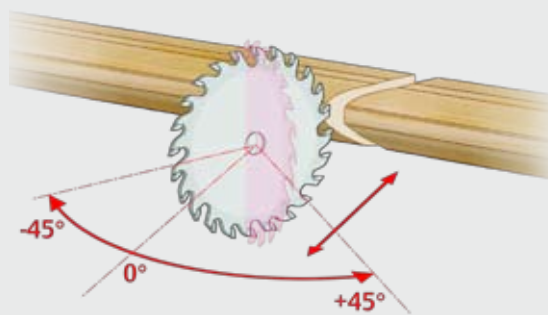
Ablängen mit jedem Winkel innerhalb +/- 45°
